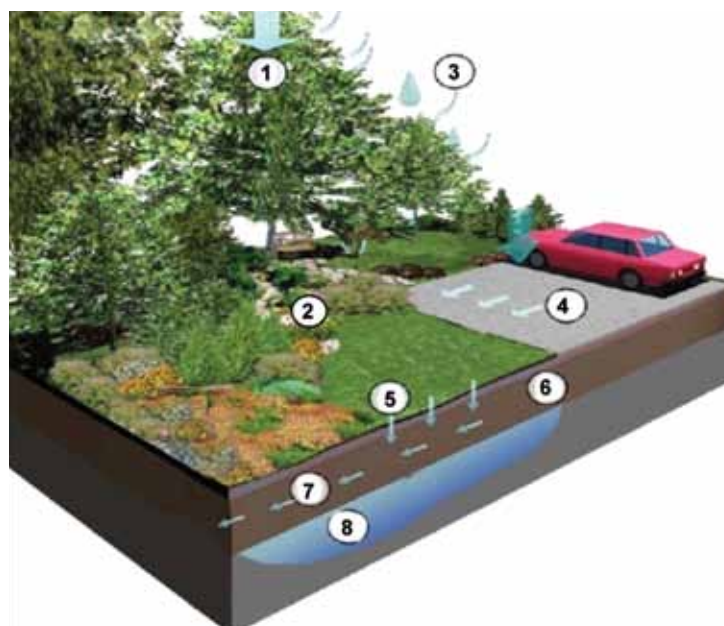
Figure 8 : Les différentes variables hydrologiques dans le concept d'«aménagement paysager absorbant» (Absorbent landscape, d'après les documents du Greater Vancouver Regional District)
